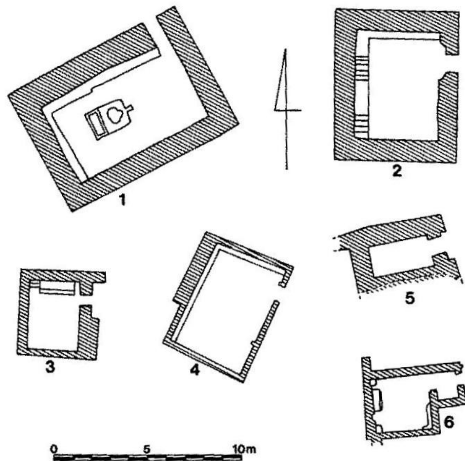
Ryc. 90. Plany świątyń z dorzecza Chaburu, przełom okresu wczesnodynastycznego II i III: 1 – Tell Brak, 2 – Tell Kaszkaszuk, 3 – Tell ar-Raqai, 4 – Tell Atidz, 5 – Tell Czagar Bazar, 6 – Tell Chuera (wg Matthews R. J. 2002, 187, fig.1).
