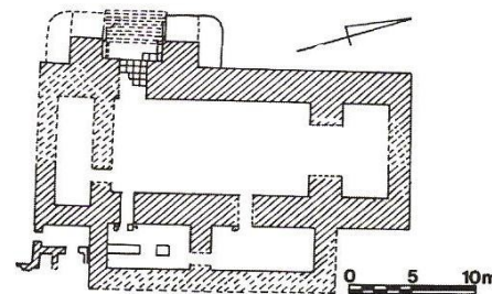
Ryc. 92. Aszur, plan świątyni Ishtar (warstwa E, wg Andrae W. 1977, 112, fig. 89).
