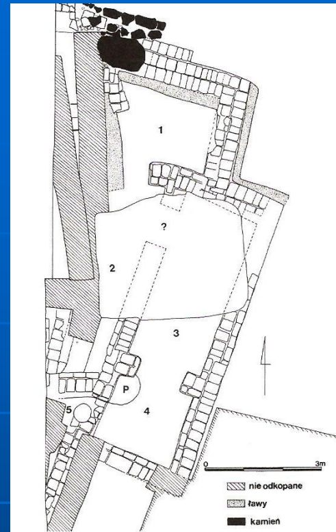
Ryc. 91. Tell Arbid, plan świątyni we wschodniej dzielnicy. Początek okresu wczesnodynastycznego III. Rys. M. Momot, D. Ławecka. P – palenisko.
