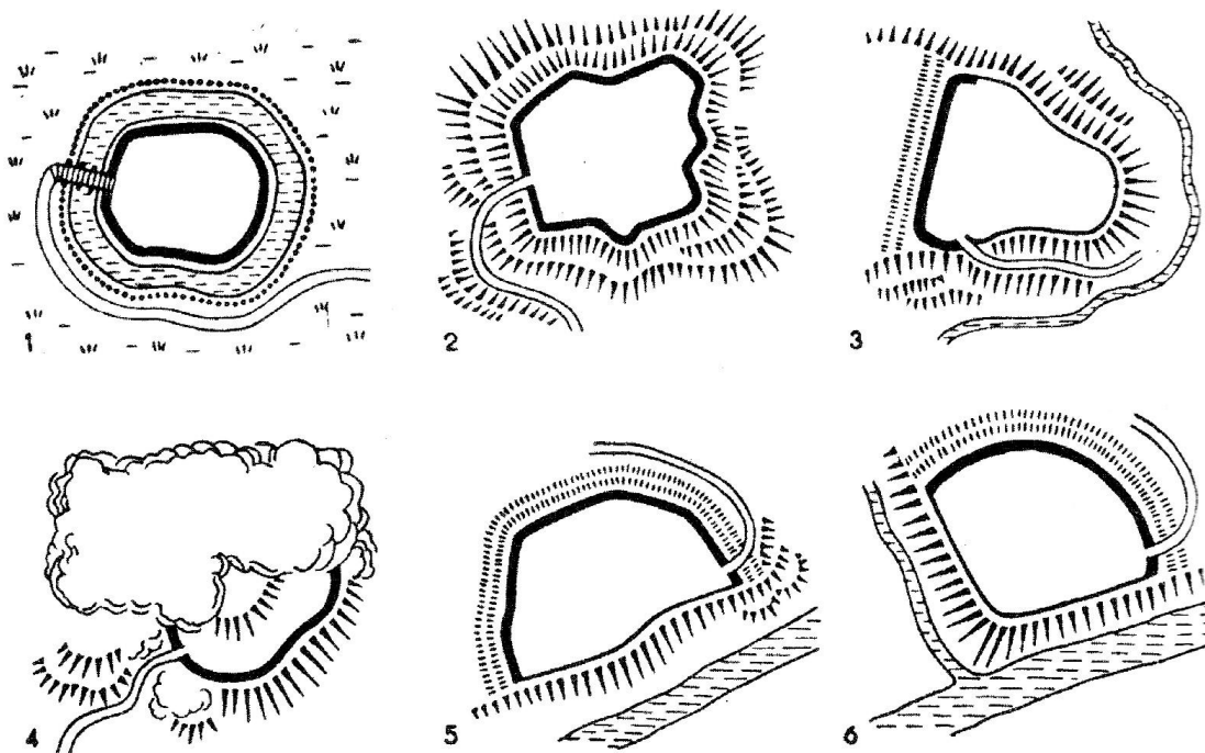
Obr. 7. 2. Geomorfologické typy polohy hradišť. 1: blatné hradiště, 2: na vrcholu kopce (stolové hory), 3: na ostrožně, 4: na spočinku svahu, 5: na vysoké říční terase, 6: na soutoku. Podle: Coblenz 1982. – Fig. 7.2. Geomorphological types of hill-fort location in the Bronze Age. 1: river meander (fenland, floodplain), 2: hilltop (table), 3: spur, 4: hill-side, 5: high river terrace, 6: confluence. After Coblenz 1982.
