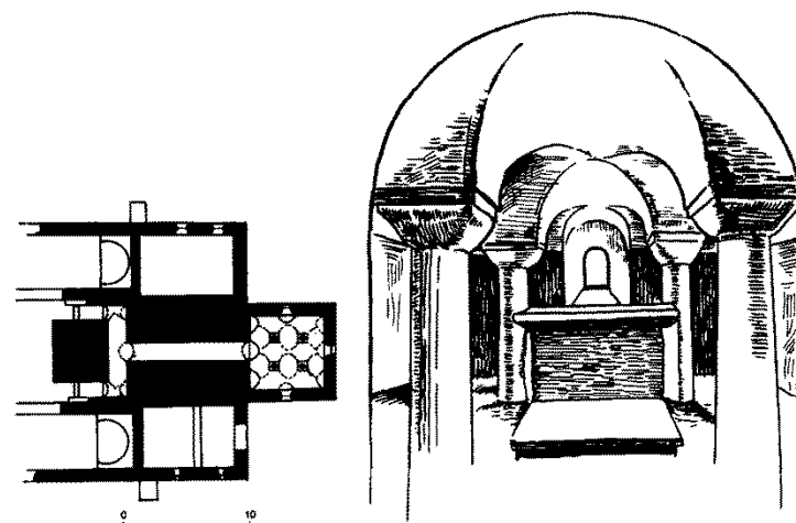
Reichenau, Oberzell, St. Georg, 896–913. Vpravo a vlevo od schodiště stoupajícího k chóru vedou schody do 2 štol, které se setkávají před stolou směřující v ose stavby k východu. Tato stola vede k raně formě halové krypty se 4 sloupy.
