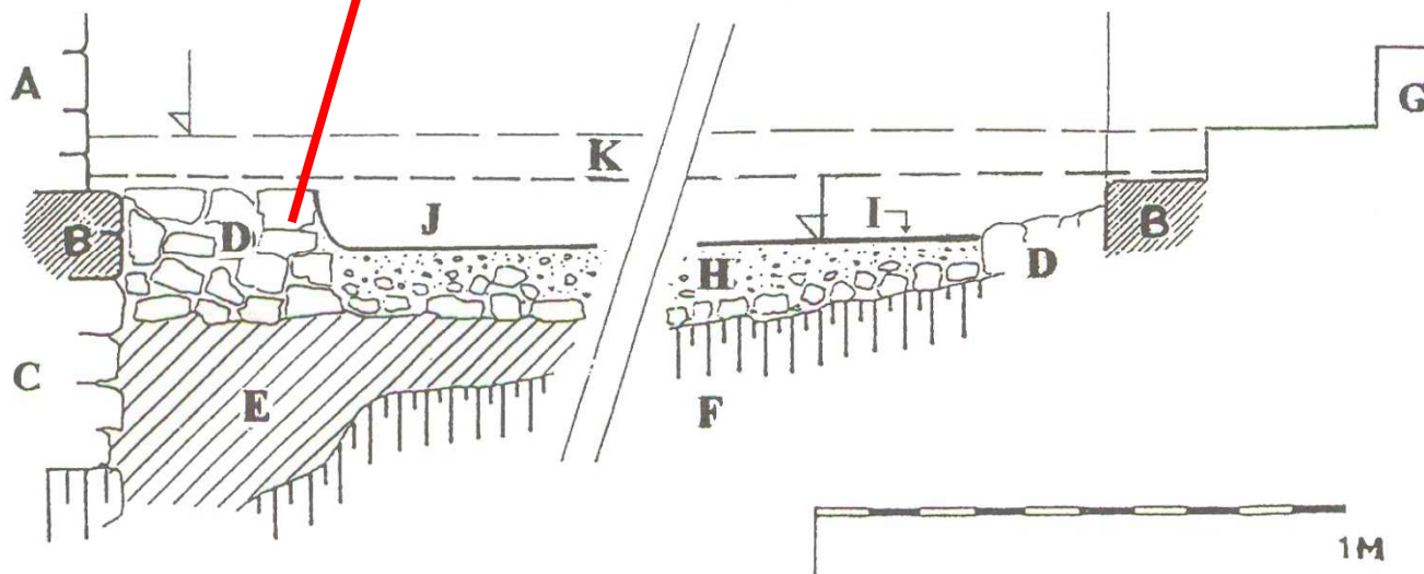
L. Konečný Znojemska rotunda – schématický řez konstrukcí podlahy při jižním a severním obvodovém zdivu lodi, podle stavebněhistorického průřezu 1989 (výkres Ing. arch. L. Kulísková)
