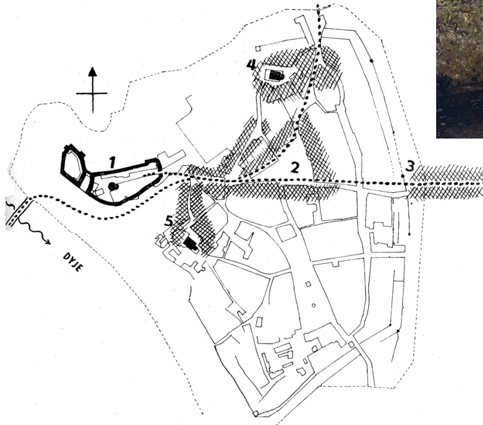
Rekonstrukce předměstské aglomerace Znojma. 1 – přemyslovský hrad s předhradím, 2 – podhradní trhová ves (marka, újezdec), 3 – Uherčice (vicus Ungarorum) a pozdější Sadovany, 4 – okrsek michalského kostela, 5 – osídlení v místech mikulášské ostrožny a pozdější Velké františkánské ulice.
