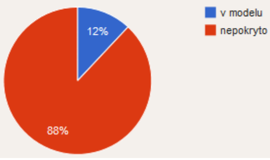
Odhad úplnosti daného modelu
