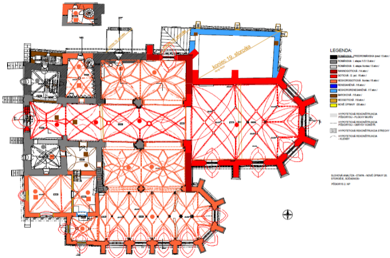
Pôdorys druhého nadzemného podlažia Katedrály sv. Martina s farebne rozlíšenými stavebnými etapami. Janovská, M. a kol.: Architektonicko-historický výskum Katedrály sv. Martina v Spišskej Kapitule.
