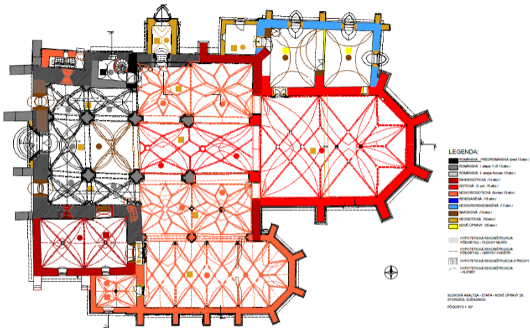
Pôdorys prízemnia Katedrály sv. Martina s farebne rozlíšenými stavebnými etapami. Janovská, M. a kol.: Architektonicko-historický výskum Katedrály sv. Martina v Spišskej Kapitule.
