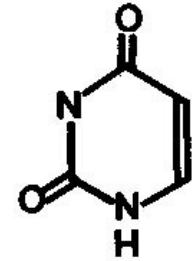
uracil
