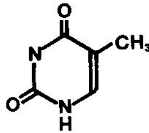
tymin
