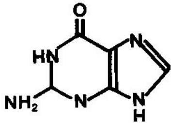
guanin
