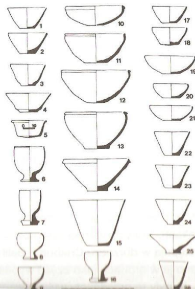
Ryc. 29. Tell Brak, ceramika z okresu wczesnodynastycznego III (wg Oates D. i in 2001, Fig. 454:1435-37, 1463, 1443-44, 1448, 1451-52; 455:12; 456:1490-94; 457:1512, 1514, 1525, 1527; 458:1528, 1530, 1539-40; 459:1543, 1549-50).
