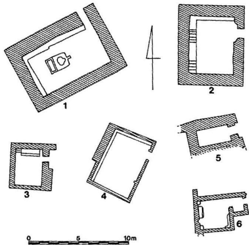
Ryc. 90. Plany świątyń z dorzecza Chaburu, przełom okresu wczesnodynastycznego II i III: 1 – Tell Brak, 2 – Tell Kaszkazuk, 3 – Tell ar-Raqai, 4 – Tell Atidz, 5 – Tell Czagar Bazar, 6 – Tell Chuera (wg Matthews R. J. 2002, 187, fig.1).
