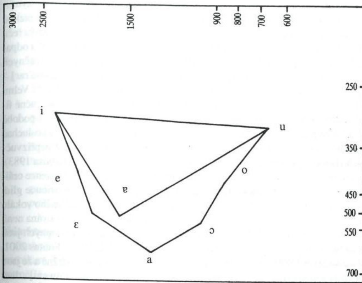
Obrázek 9: Akustický trojúhelník portugalských ústních samohlásek (podle Delgado-Martins 1988)
