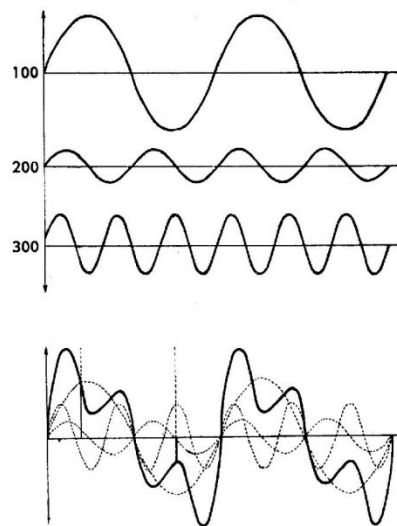
Složené tóny
