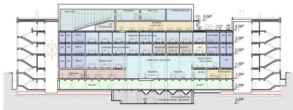
podélný řez A-A navrhovaný stav 1:250
