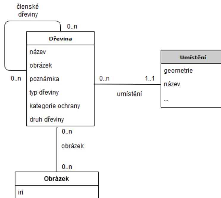
Obrázek 1 Diagram datového modelu dřevin . Šedě podbarvené části jsou specifikovány jinými otevřenými formálními normami, nebo se jedná o číselník.
