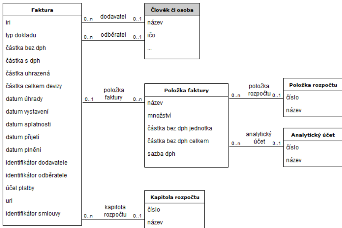
Obrázek 1 Diagram datového modelu faktur
