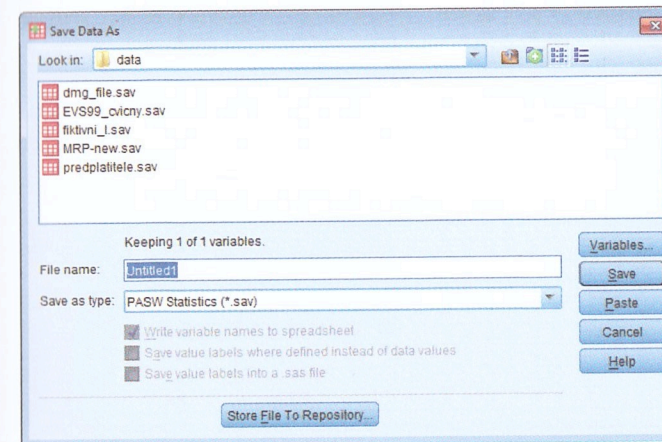
Obr. 2.13 Ukládání dat
