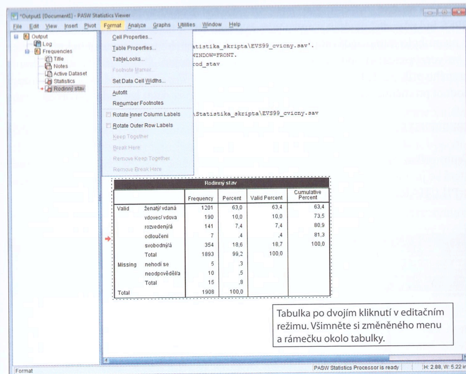
Obr. 2.4b Editace výstupu
