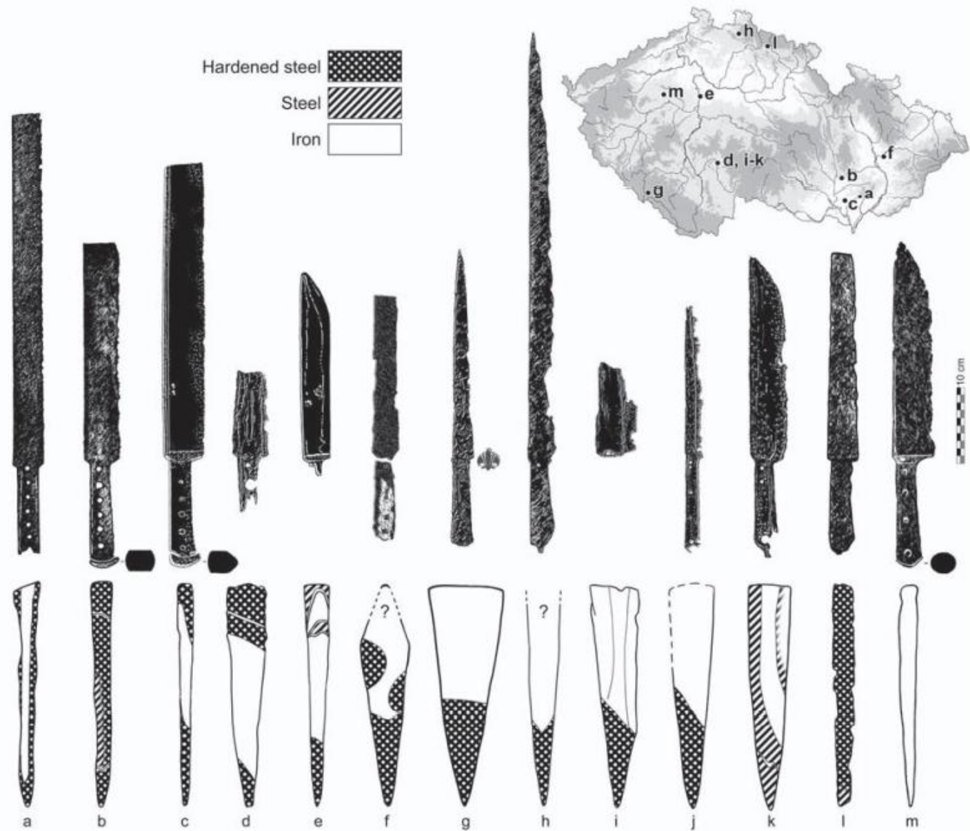
Obr. 135: Přehled metalograficky zkoumaných tesáků z území České republiky: a – Věteřov; b – Horákov; c – Bolera-dice; d – Sezimovo Ústí (698); e – Praha (650); f – Přerov; g – Horská Kvilda; h – Liberec; i – Sezimovo Ústí (697); j – Sezimovo Ústí (696); k – Sezimovo Ústí (693); l – Dolní Štěpanice; m – Krásná dolina (podle Žákovský – Hošek – Bárta 2013, obr. 15).
