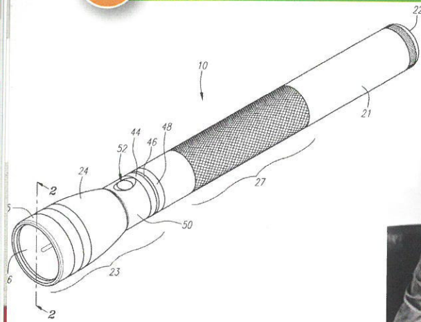
originalan nacrt svjetiljke MagLite
