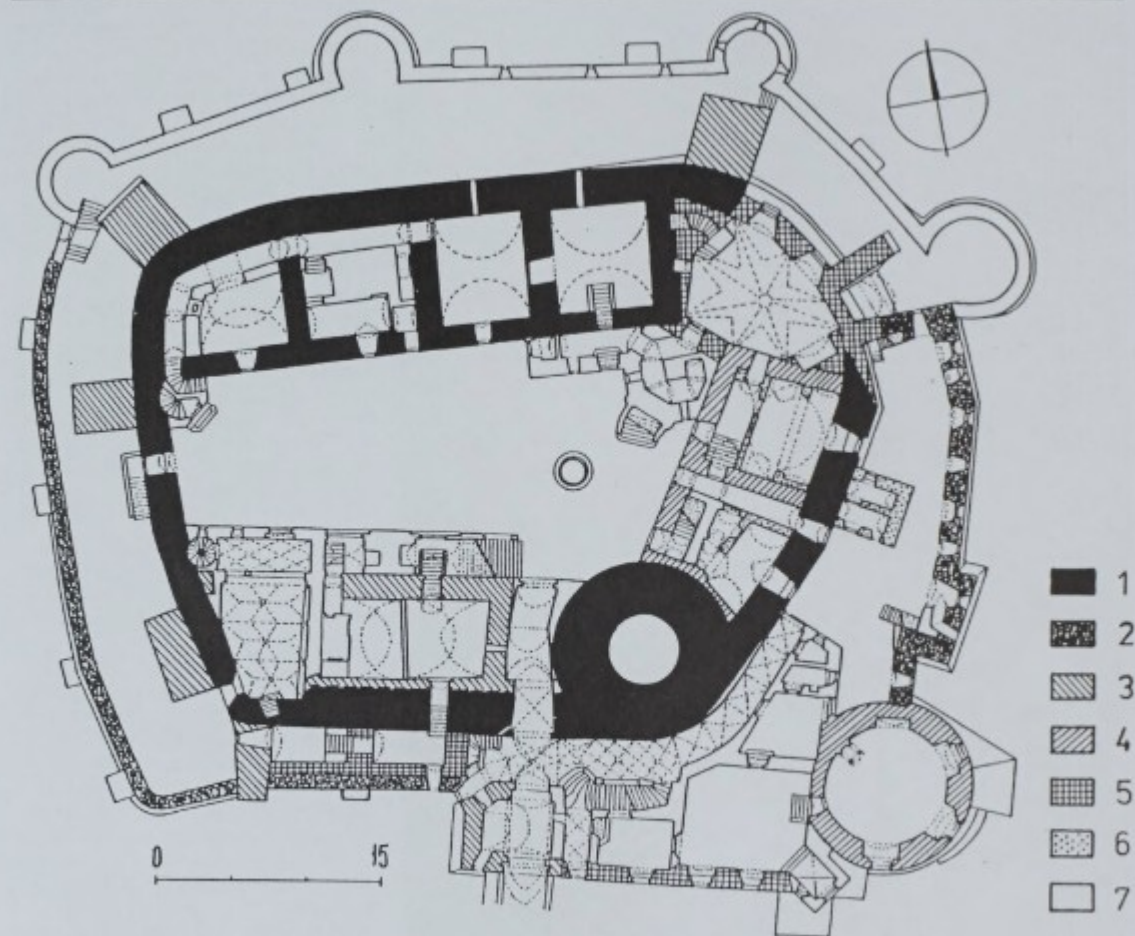
218. Bouzov – analýza půdorysu hradního jádra. 1 – jádro z počátku 14. století, 2 – využití zdivo parkánu, 3 – konec 14. století nebo konec druhé třetiny 15. století, 4 – přelom 15. a 16. století, 5 – renesance, 6 – barok, 7 – produkty reorganizace (některé budovy jsou téhož původu, ale stojí na starších základech – jižní a z velké části i severní palác).
