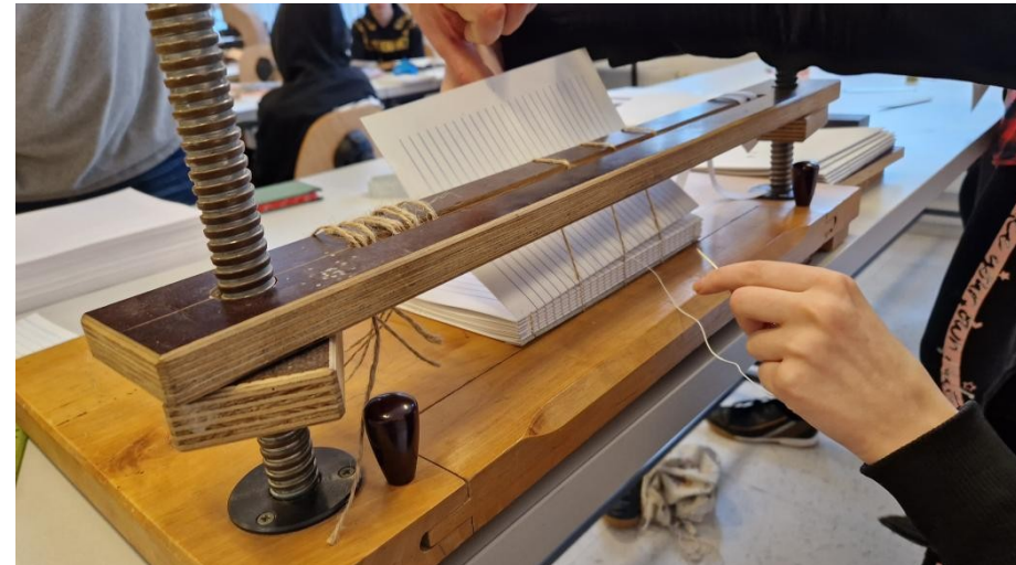
Knihářský stávek - našívání složek na vazy
