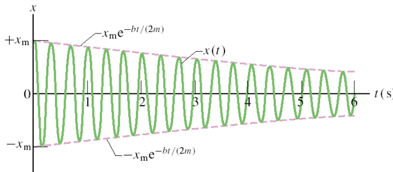
Časový průběh slabě tlumených kmitů
