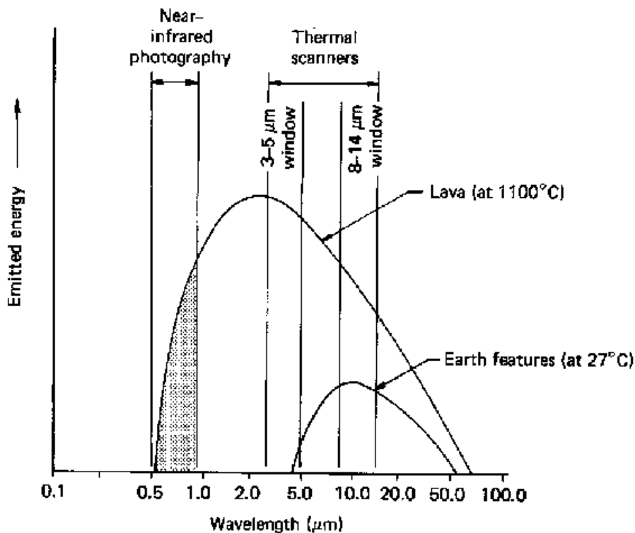
Obr. 2.7 Intenzita vyzařování objektů s běžnou teplotou a objektů výrazně horkých v blízké infračervené části spektra
