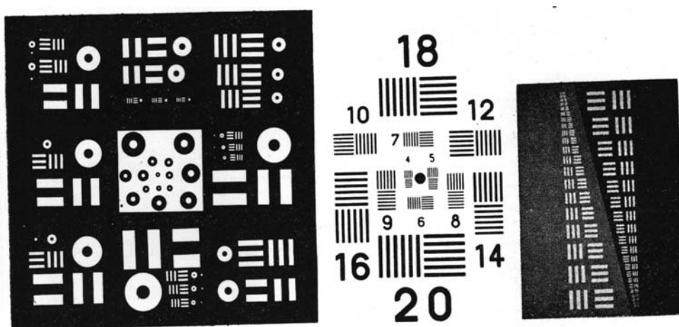
Obr. 2.8 Vzorníky pro určování rozlišovací schopnosti snímků
