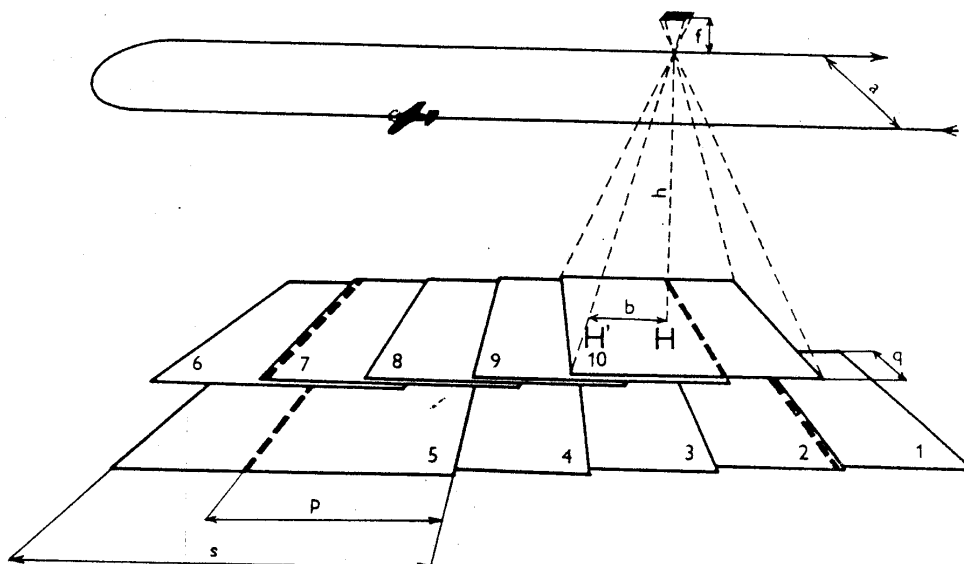
Obr. 3.7b Schéma řadového snímkování, základní druhy překryvů
