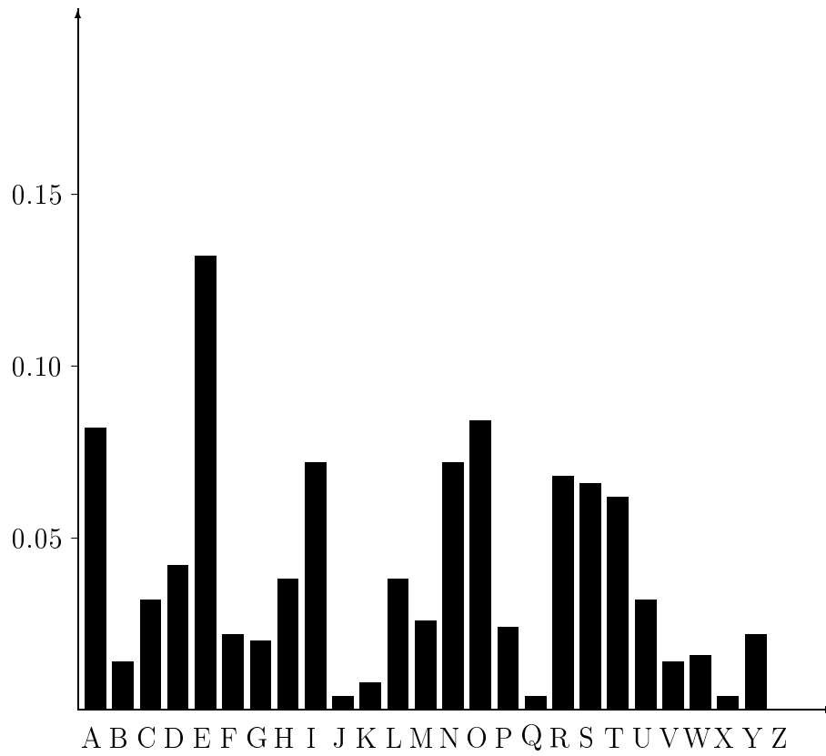
Obrázek C.1: Histogram četností písmen anglického jazyka
