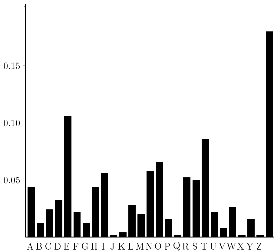
Obrázek B.1: Histogram četností písmen českého jazyka (s mezerou)
