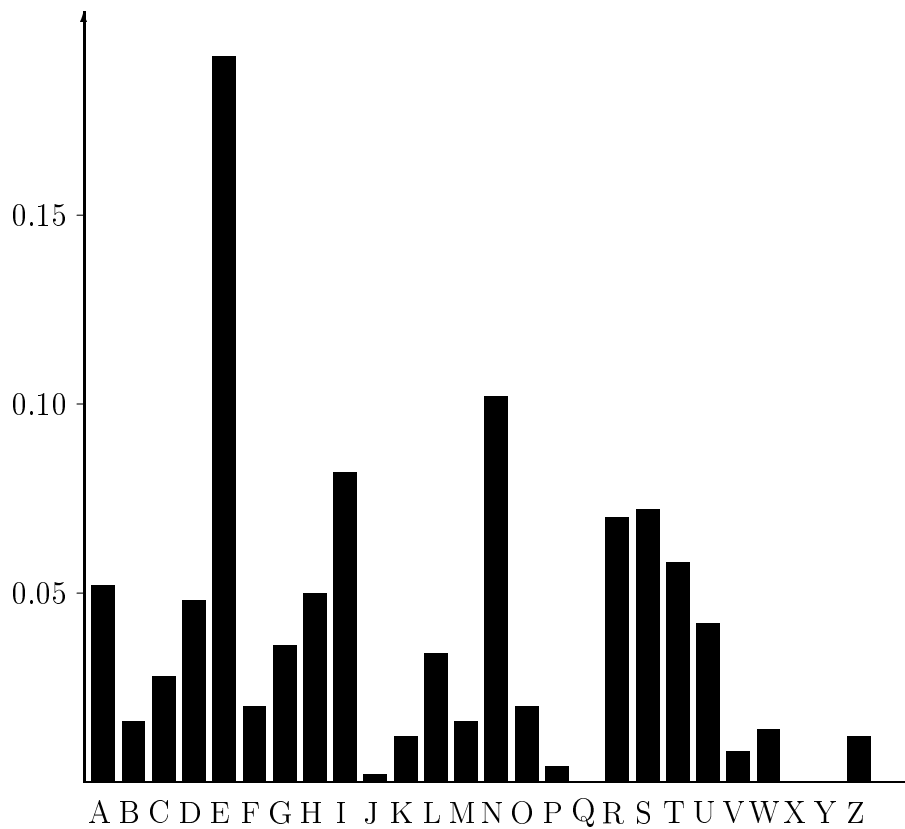
Obrázek D.1: Histogram četností písmen německého jazyka
