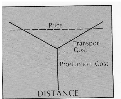
Obr. 11: Systém „c.i.f.“
