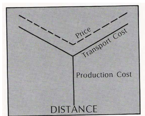
Obr. 12: Systém „f.o.b.“
