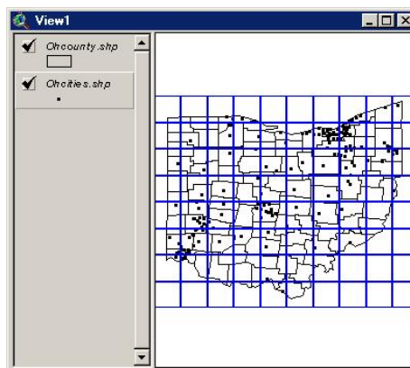
Obr. 2.4 Analýza kvadrátů – pravidelné rozmístění buněk
