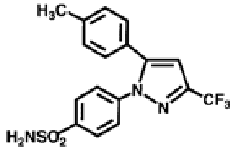
Celecoxib
