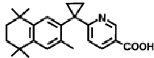
LG 100268
