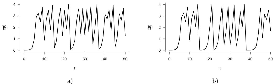
Obrázek 1.9: Graf posloupnosti x(t) generované modelem x(t+1) = x(t)(4 + x(t)) s počáteční hodnotou a) x(0) = 0,001 a b) x(0) = 0,001001
