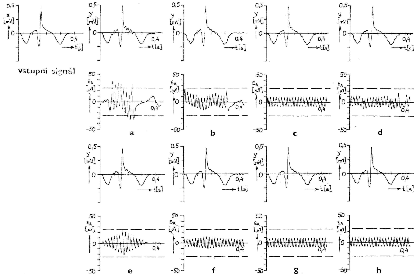
Obr. 4. Ukázky zesílení užitečného signálu vlivem různých typů úzkopásmových zádrží — a) výstup filtru H_{8,5}^{(1)} , b) výstup H_{16,5}^{(1)} , c) výstup H_{22,5}^{(1)} — systému s optimální hodnotou K = 22 pro délku periody signálu 110 vzorků, d) výstup H_{24,5}^{(1)} , e) výstup H_{8,5}^{(2)} , f) výstup H_{16,5}^{(2)} , g) výstup H_{22,5}^{(2)} — optimálního systému, h) výstup H_{24,5}^{(2)} f)_{vz} = 250 Hz, kvantovací krok 1 \mu\text{V} )
