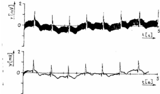
Obr.2-31 Filtrace reálného signálu EKG s obsahem síťového rušení Lyapunov pásmovou zádrží s K=12 , p=5
