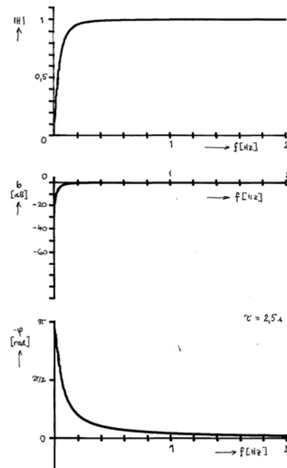
Obr.2-26 Frekvenční charakteristiky pasivního RC člunku používaného dříve na vstupu elektrokardiografů
