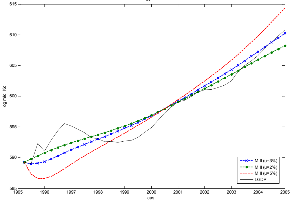
Model II - zmeny g_{ss} - odhady potencialu
