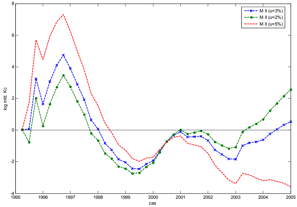
Model II - zmeny g_{ss} - mezera vystupu
