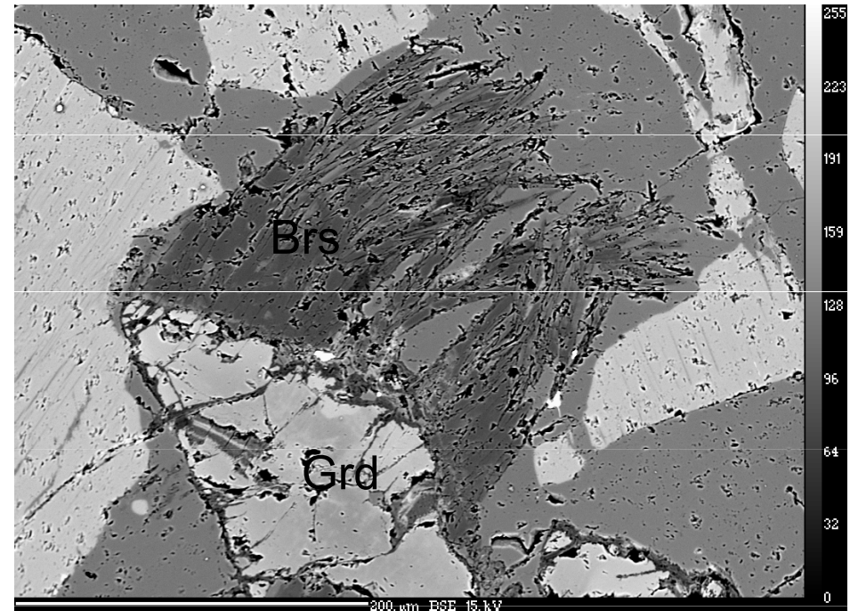
Boralsilit na grandidieritu, Horní Bory
