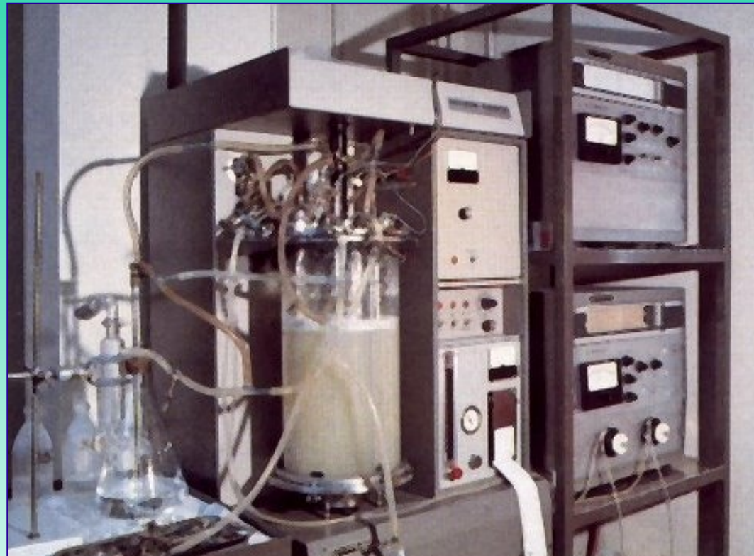
laboratorní bioreaktor
