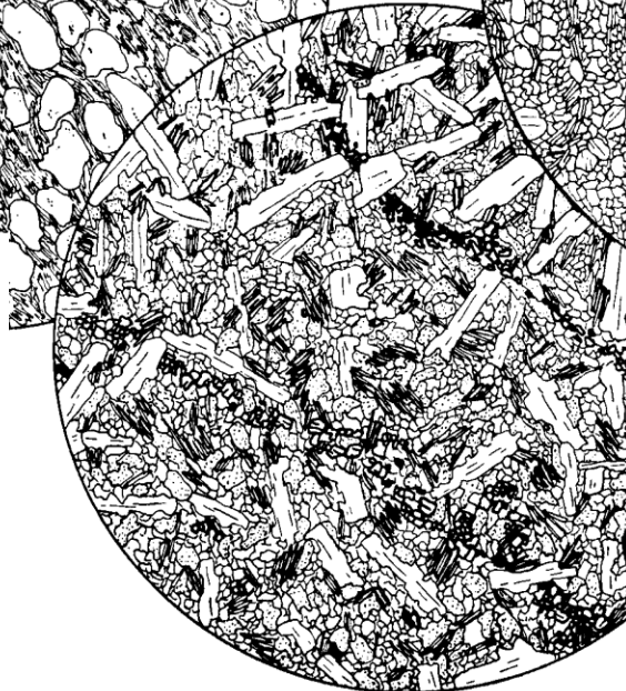
B) blastoofitická struktura: Zelená břidlice, Kralupy nad Vltavou. Reliktně zachovaný tvar a uspořádání lišt původně bazických, nyní kyselých plagioklasů v rekrytalované základní tkáni složené z drobného albitu, chloritu, křemene a titanitu, vytvářejícího proužky.
