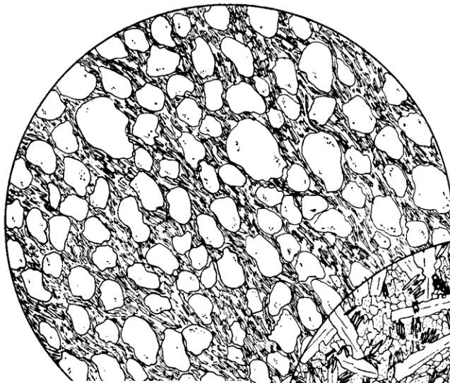
A) blastopsamitická struktura: Kontaktně metamorfovaný algonkický pískovec, Koupě u Hudčic. Reliktní klastická zrna křemene uložená v jemnozrnné rekrytalované základní tkáni, která se skládá z jemných šupinek biotitu a zrněk křemene.
