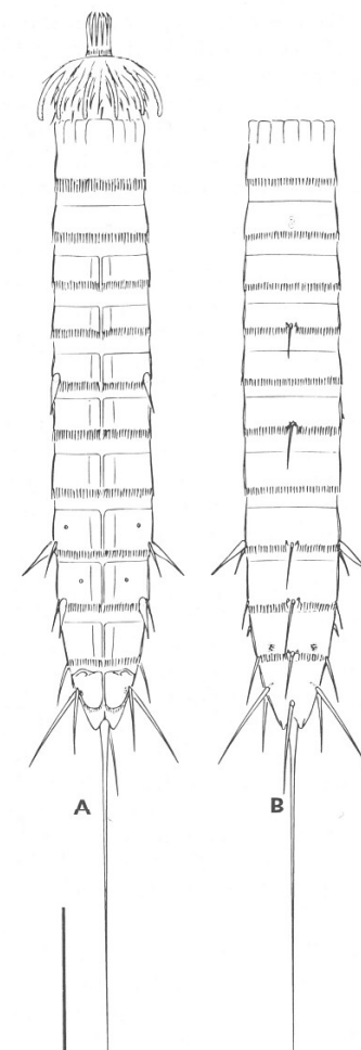
Zelinkaderes floridensis (Cyclorhagida), samice: A - introvert vychlípěn, břišní strana; B - introvert zatažen, uzavřen 2. zonitem, hřbetní strana; měříko 100 \mu m
