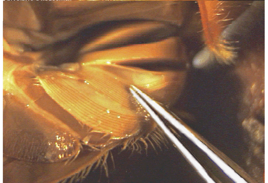
Lupenitá končetina opisthosomatu s funkcí žaber
