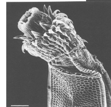
Přída larvy Halicryptus spinulosus (měřítko 100 μm), Baltské moře.
