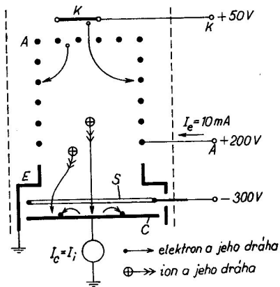
Obr. 5.51. Schuermannův vakuometr s potenciálovou bariérou A – mřížková anoda; K – katoda; C – kolektor; E – stínění; S – prstencová elektroda (supresor)
