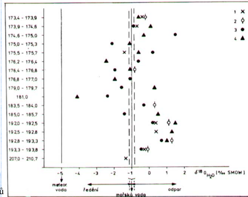
HV-301 Čejkovice. Graf \delta^{18}\text{O}_{\text{H}_2\text{O}} HLADÍKOVÁ (1985). Převzato z práce HLADÍKOVÉ (1988). 1- Pirenella, 2- Cerastoderma, 3- Nematorella, 4- Congeria.
