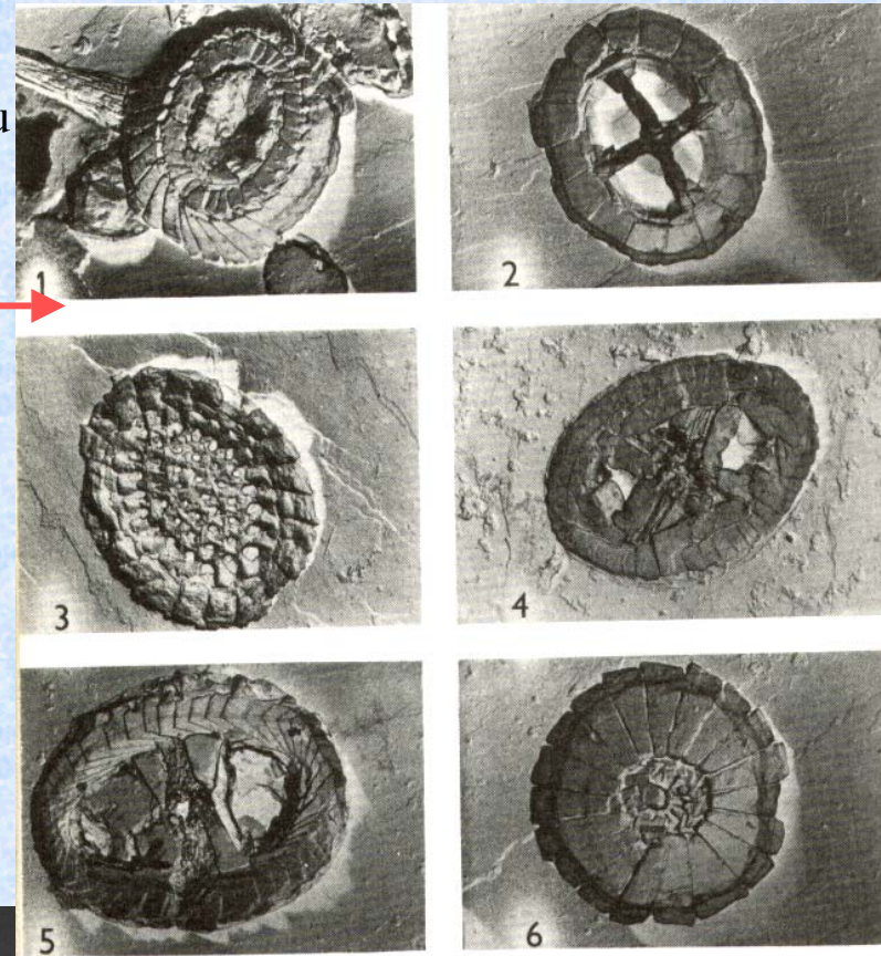
Vápenatý nanoplankton, svrchní křída, Kystra (snímky zhotovené pomocí transmisního elektronového mikroskopu): 1 Watznaueria barnesae , 2 Prediscosphaera propinqua , 3 Cribrosphaerella ehrenbergi , 4 Eiffellithus trabeculatus , 5 Tranolithus exiguus , 6 Biscutum rotarium
