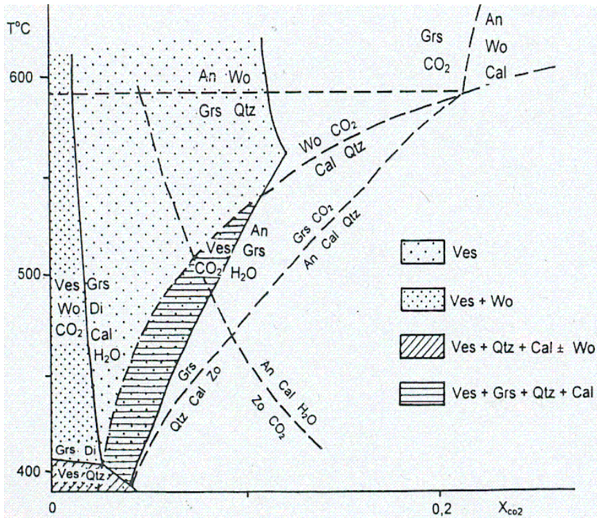
Obr. 1. Schematický T - X CO2 diagram vybraných reakcí v systému CMAS-H 2 O-CO 2 při P fluid = P celk. = 200 MPa (upraveno podle Valleyho et al. 1985 a Labotky et al. 1988) Fig. 1. Schematic T - X CO2 diagram showing selected reactions in the system CMAS-H 2 O-CO 2 at P fluid = P total = 200 MPa (modified from Valley et al. 1985 and Labotka et al. 1988).
