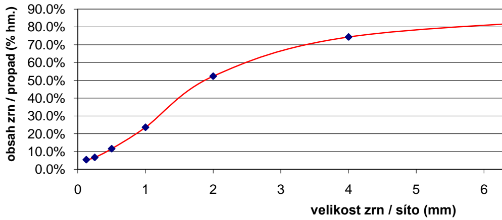
Zrnitostní křivka (Suchdol vz-8)
