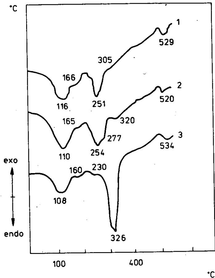
Obr. 12.18. DTA krivky: 1 — ľudských vlasov, 2 — mohérovej vlny, 3 — vlákien prírodného hodvábu v dusíkatej atmosfére (Schwenker a Dusenbury 1960).
