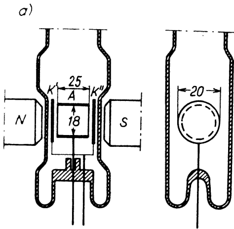
Výbojový manometr - Penning
