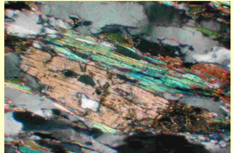
muskovit-biotitický svor se staurolitem a granátem
