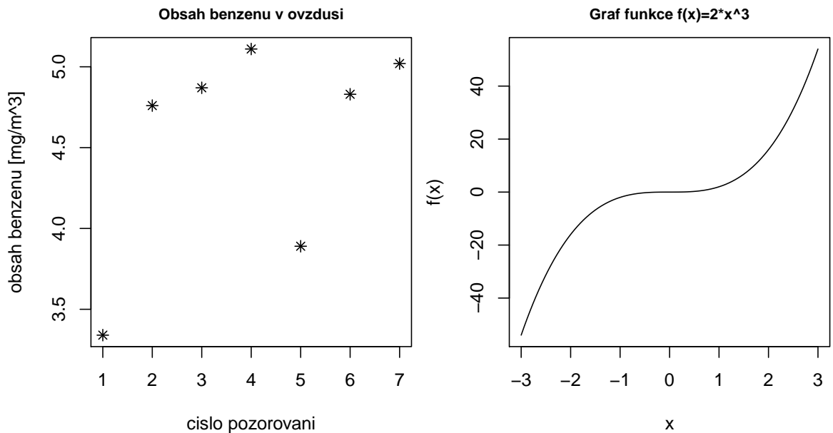
Obr. 8.1. Funkce plot()
