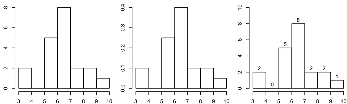
Obr. 8.6. Sklizňová ztráta obilí [g/m 3 ], zobrazení absolutních a relativních četností
