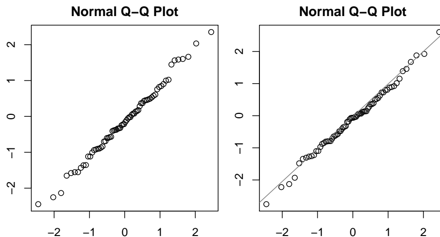
Obr. 8.11. Q-Q plot pro výběr z normálního rozložení
