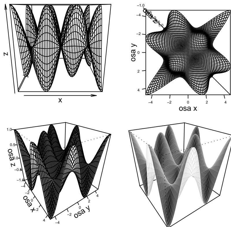
Obr. 8.14. Funkce persp()
