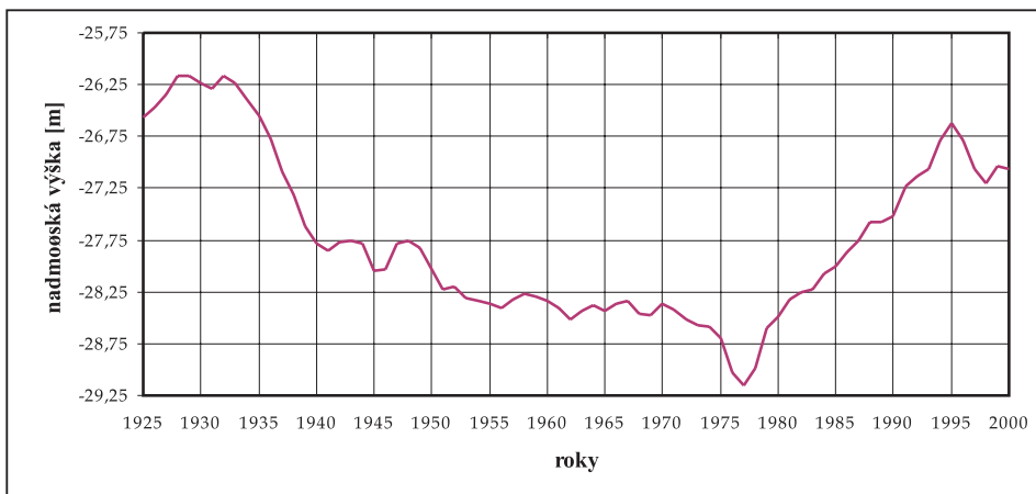
Obr. 1 – Kolísání úrovně hladiny Kaspického moře v průběhu let 1925–2000. Osa x – roky, osa y – nadmořská výška (m). Upraveno podle: Golubtsov, Lee 2000a.
