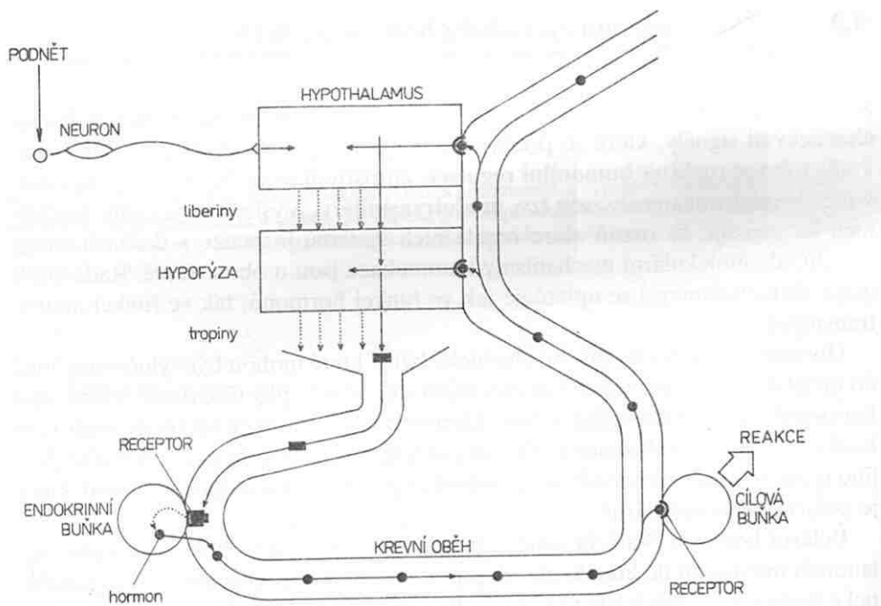
Obr. 202 Schéma endokrinní soustavy
