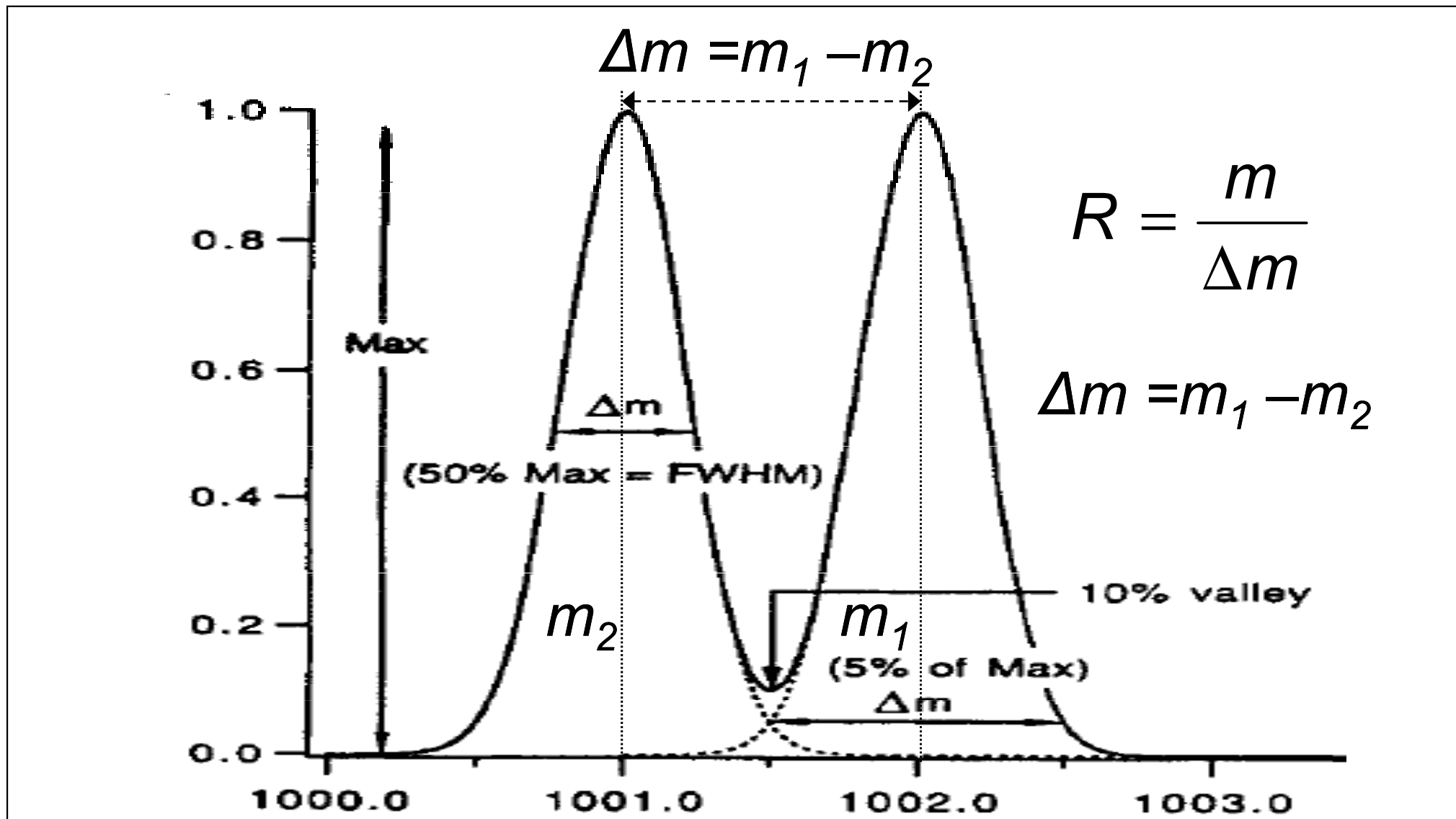
Obr. 3 Definice rozlišovací schopnosti pomocí dvou signálů m_1 , m_2 stejné velikosti, pomocí \Delta m jediného signálu při 5 % výšky maxima a \Delta m jediného signálu při 50 % výšky maxima
