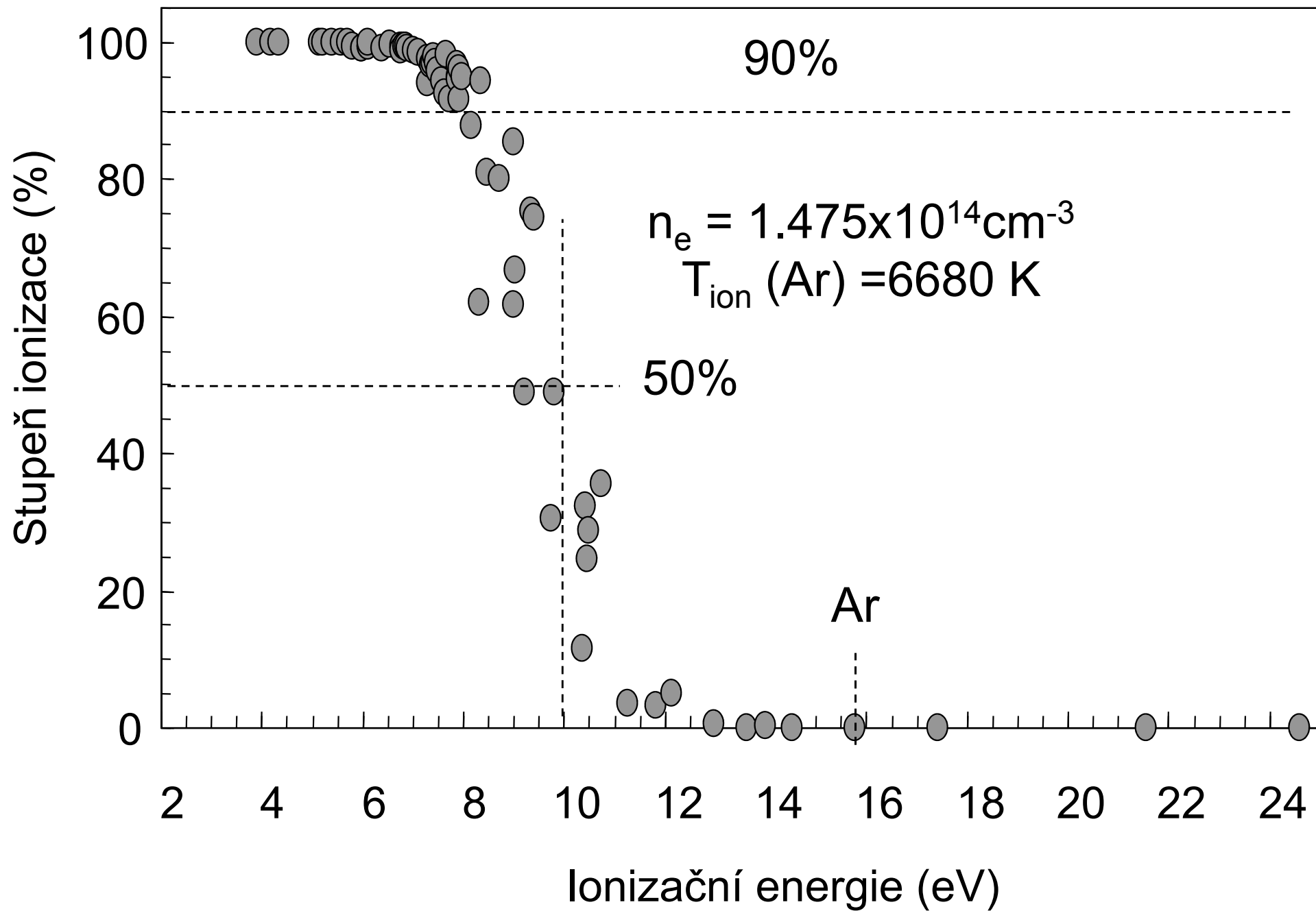
Obr. 1 Závislost stupně ionizace na ionizační energii
