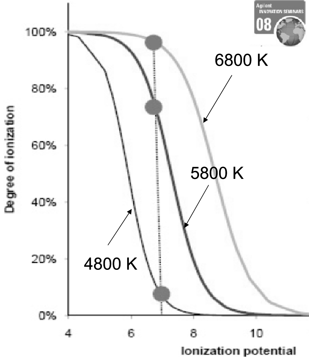
Obr. 2 Závislost stupně ionizace na teplotě
