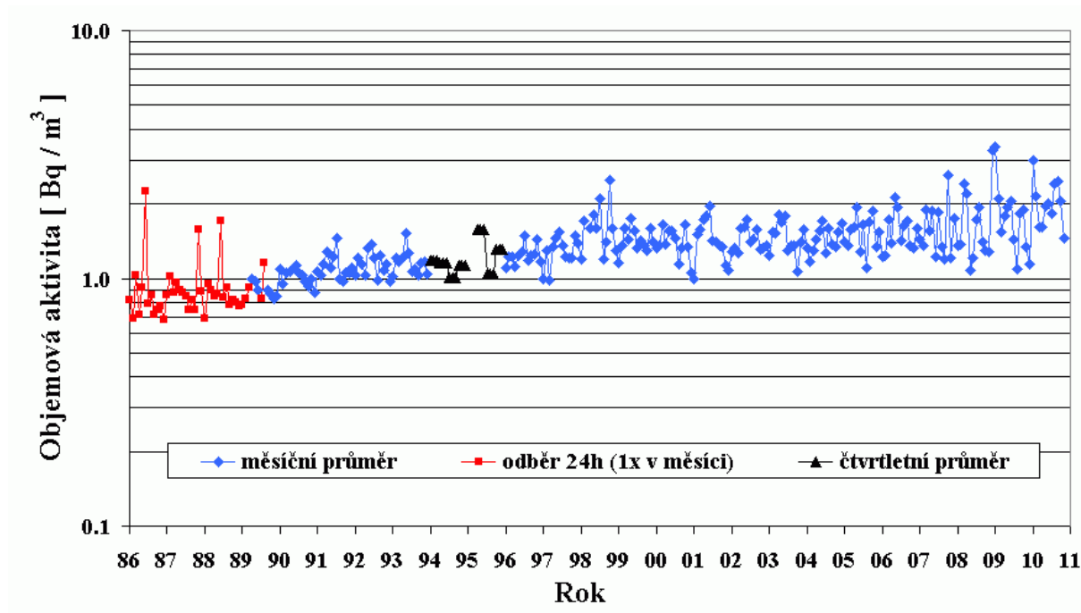
Průměrné měsíční hodnoty objemové aktivity ^{85}\text{Kr} v ovzduší v Praze http://www.suro.cz/cz/rms/ovzdusi/mesic
