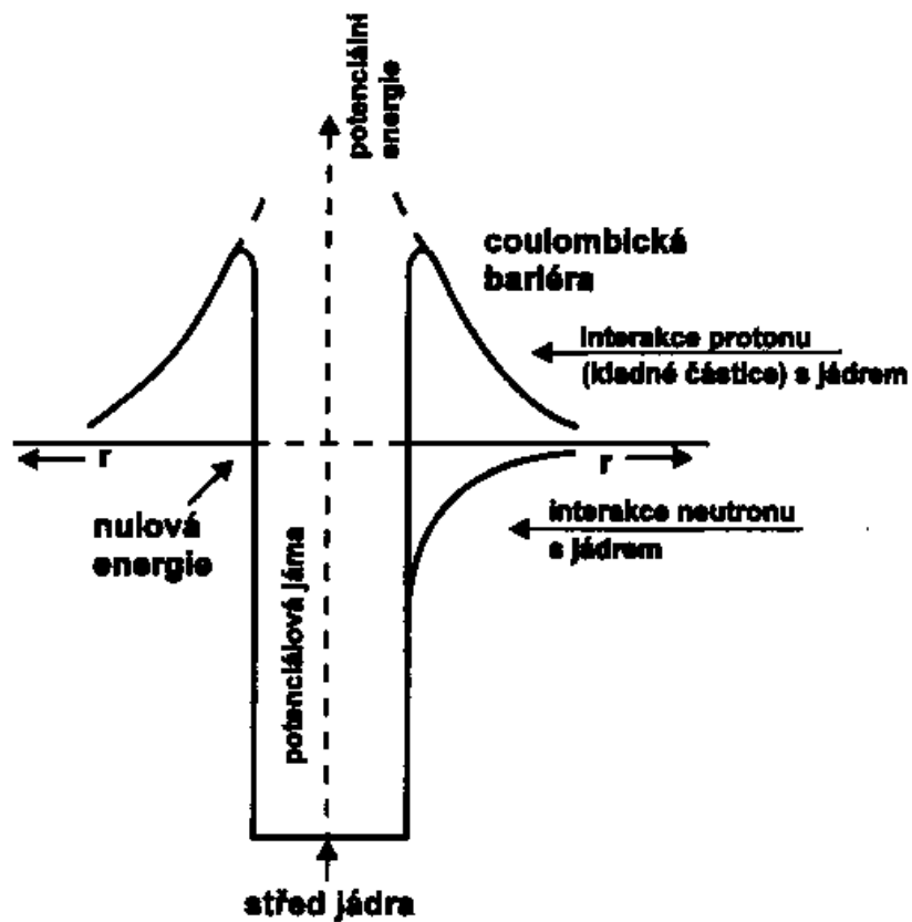
Obrázek 2: Potenciální energie při interakci jádra s nukleony.
