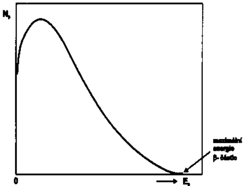
Obrázek 12: Energetické spektrum \beta_- částic.
