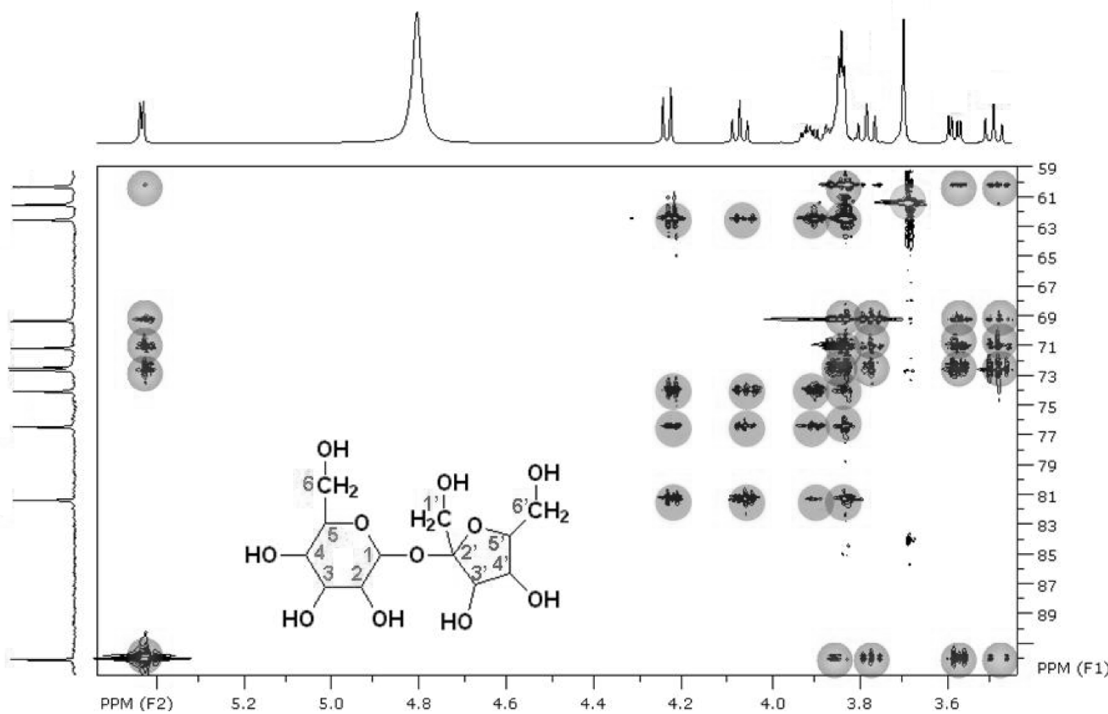
Obrázek 3: ^1\text{H} - ^{13}\text{C} HSQC-TOCSY - disacharid
