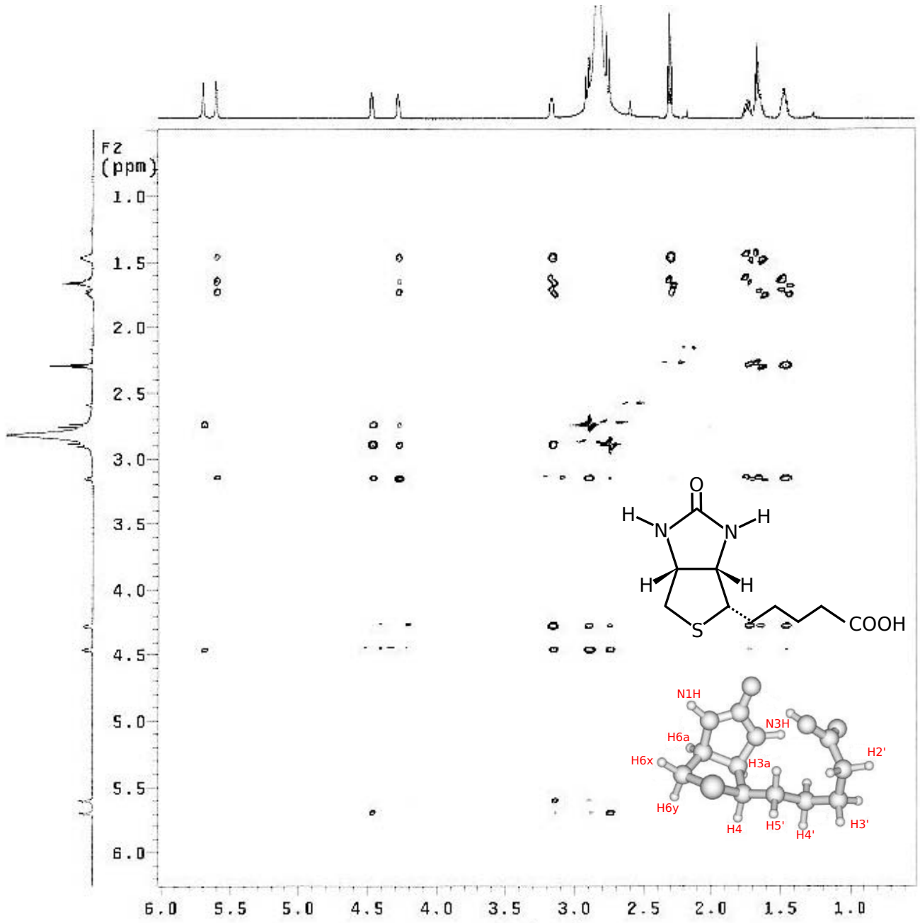
Obrázek 2: ROESY - biotin
