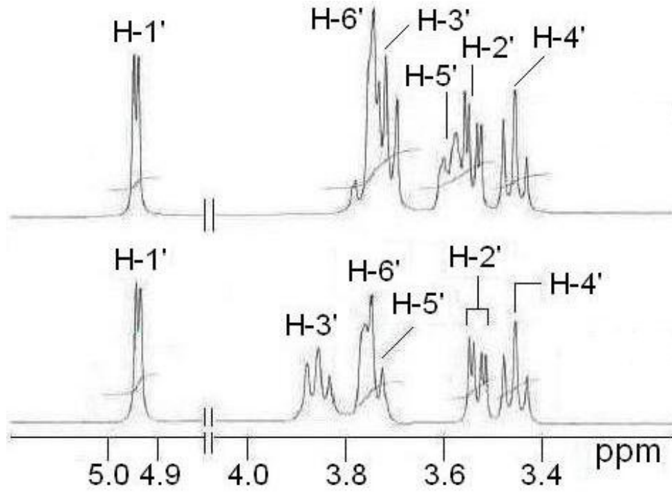
Obrázek 6: 1D ^1\text{H} - cyklodextrinová část
