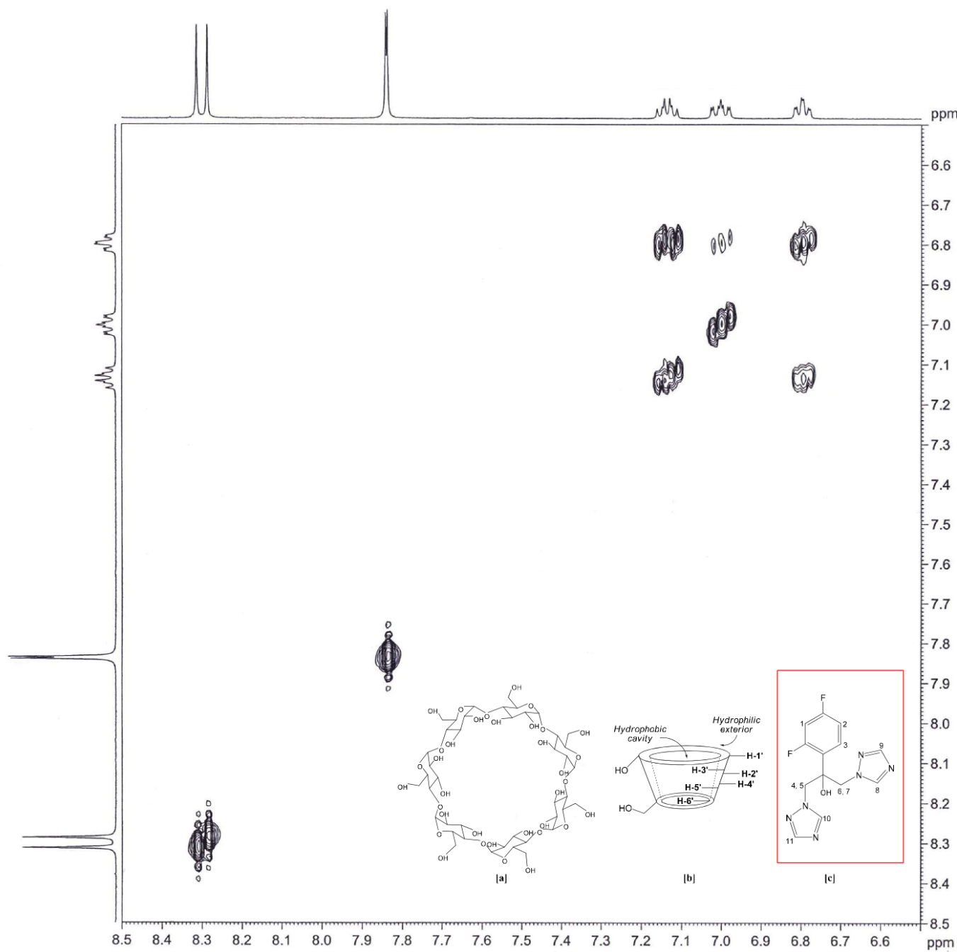
Obrázek 4: COSY - ligand
