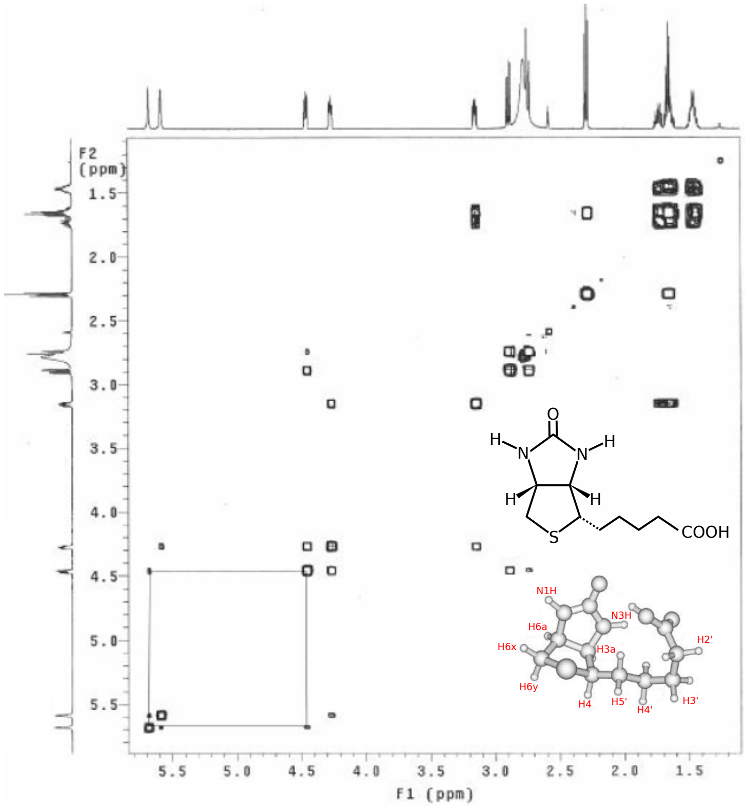
Obrázek 1: COSY - biotin
