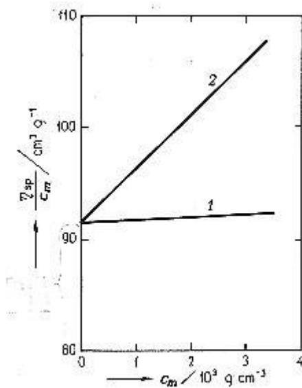
Obr. 89 Viskozimetrické údaje pro poly-L-prolin v propionové kyselině vynesené podle Hugginsovy (2) a Kraemrovoy (1) rovnice
