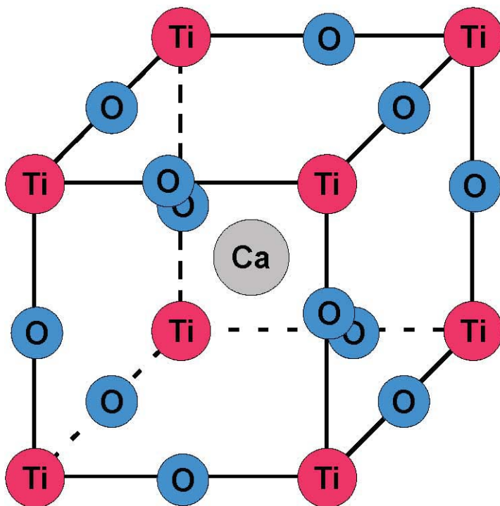
Obr. 12 Perovskitová struktura
