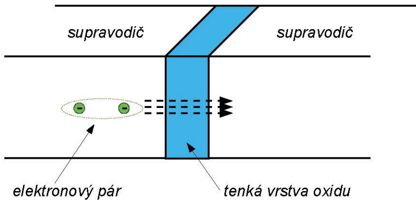
Obr. 11 Josephsonův efekt
