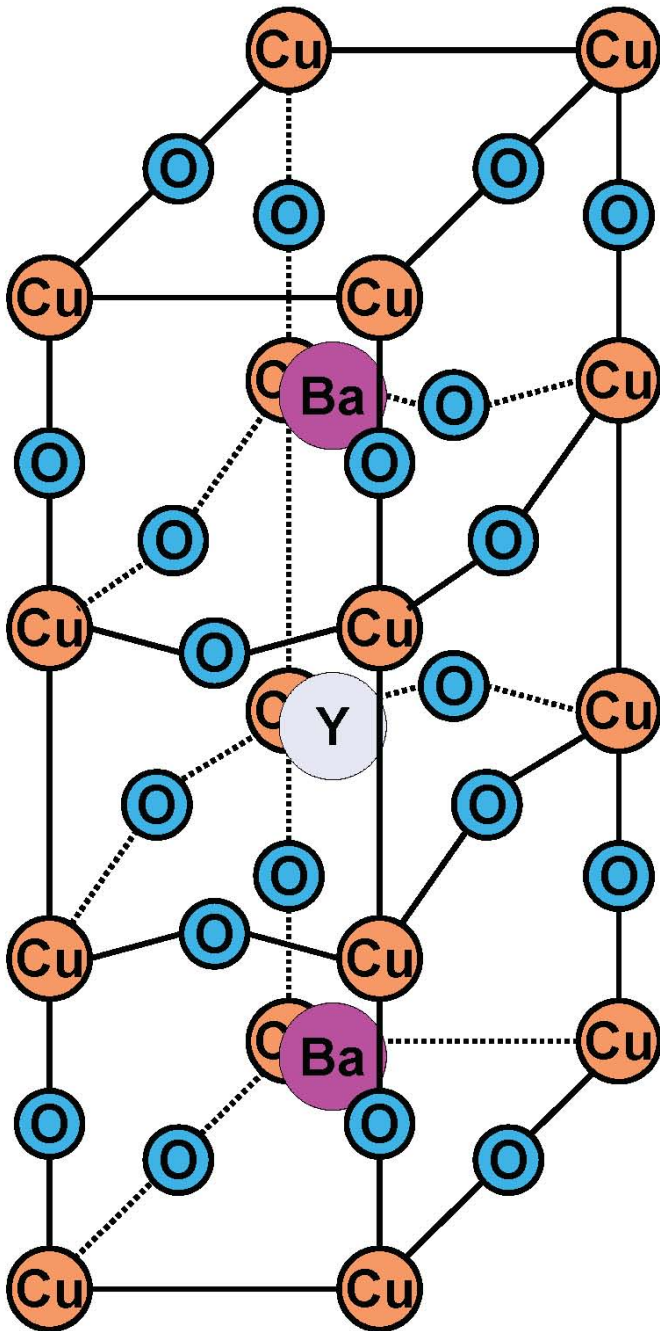
Obr. 13 Struktura YBCO supravodiče
