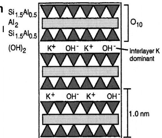
illite
