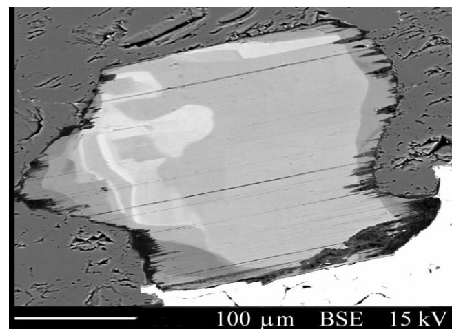
Muskovit, Bobručka
