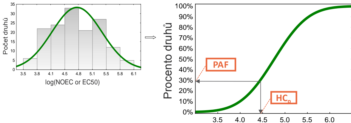
Obr. 3. Zobrazení SSD jako kumulativní distribuční funkce a odvození PAF (Potentially Affected Fraction) a HC_p (Hazard Concentration for p percent of species).
