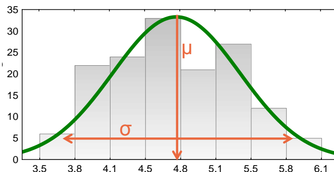
Obr. 2. Parametry normálního (Gaussova) rozložení
