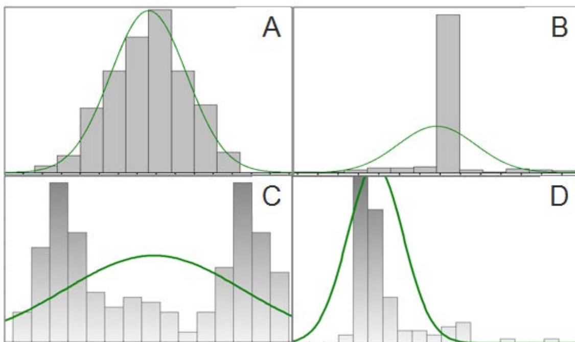
Obr. 5. Normální rozložení (zelená křivka) versus rozložení dat (šedé sloupce):
